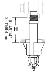
Type 3 Extended Escutcheon Tiefe Rosette Rosace encastrée
