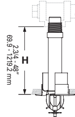
Type 2 Recessed Escutcheon Versenkte Rosette Rosace rallongée
